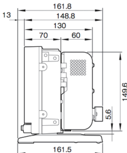
側面
