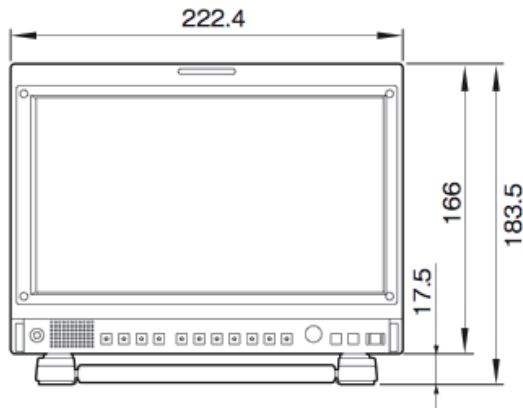
前面
