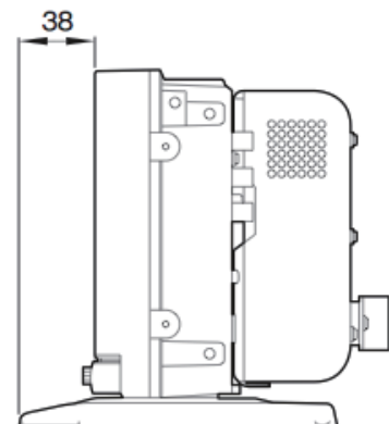
側面 (スタンド取り付けネジ位置B、C使用時)
